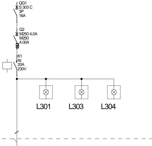
Rys.2. Schemat obwodu głównego.
